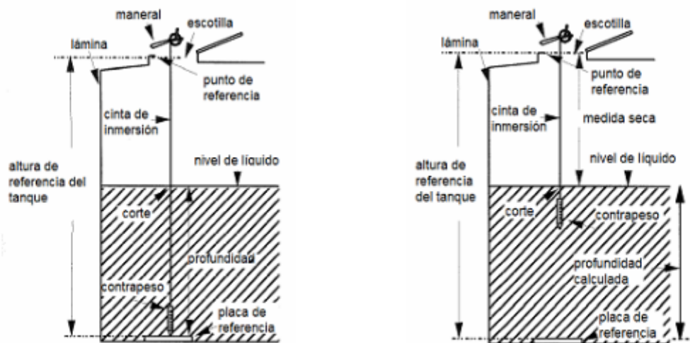
a) Medición de nivel por inmersión.
